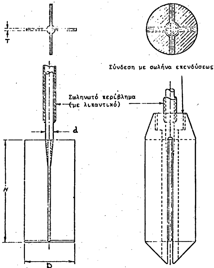
Σχήμα 2. Πτερύγιο και στέλεχος. Σχήμα 3. Προστατευτική θήκη πτερυγίου.
