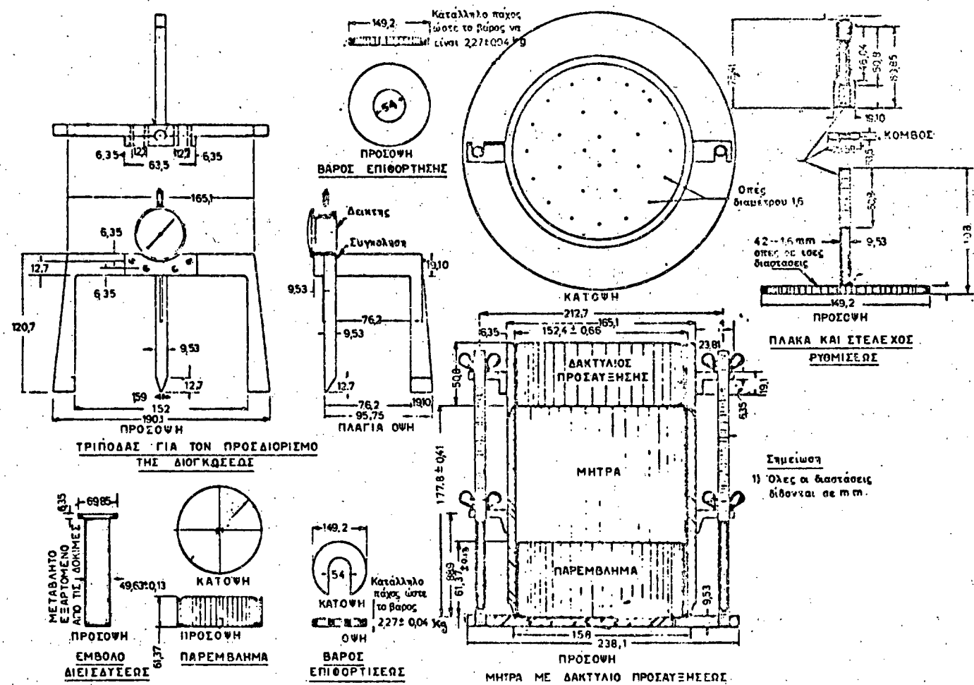
Σχήμα 1. Συσκευή δοκιμής Καλιφορνιακού Λόγου Φέρουσας Ικανότητας.
