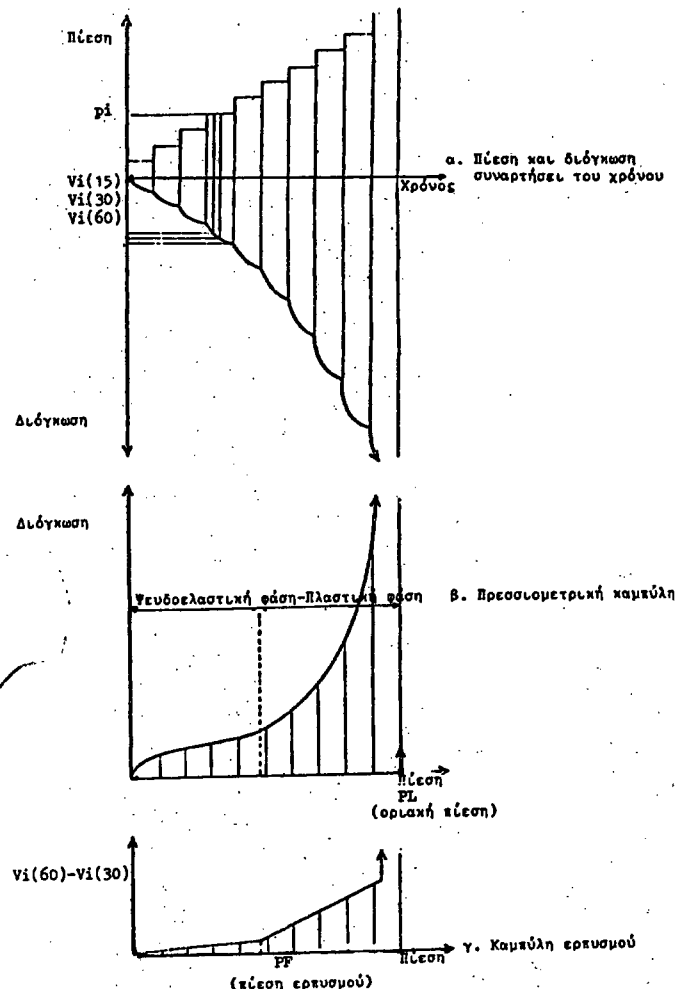
ΣΧΗΜΑ 2. Διαγράμματα πρεσσιομετρικής δοκιμής
