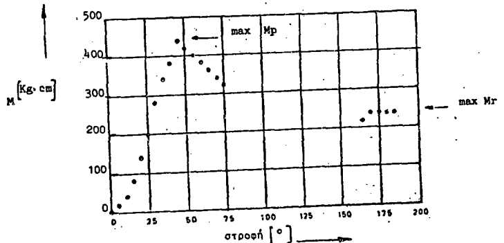
Σχήμα 4. Διάγραμμα μεταβολής στρεπτικής ροπής σε συνάρτηση με τη γωνία στροφής.
