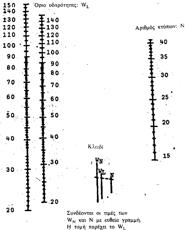
Σχήμα 2. Νομογράφημα προσδιορισμού ορίου υδαρότητας.
