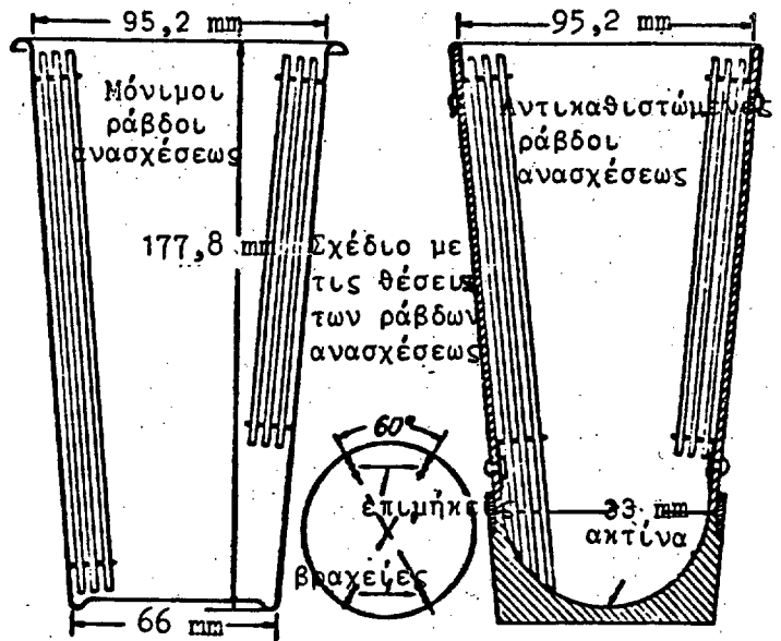
Σχήμα 1. Κύπελλα διασποράς.
