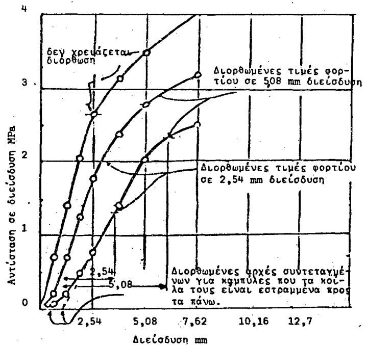
Σχ. 1. Διόρθωση καμπυλών τάσεων-παραμορφώσεων.
