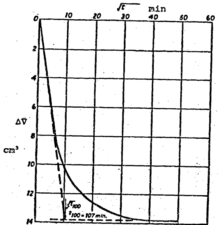
Σχήμα 1 Σχέση μεταβολής του όγκου - √t κατά τη διάρκεια στερεοποίησης σε πλευρική ομοιόμορφη τάση σ 3 .
