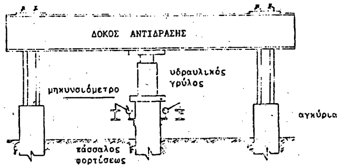
Σχ. 1. Διάταξη επιβολής φορτίου σε πάσσαλο με γρύλο και με σύστημα αγκυρώσεως.
