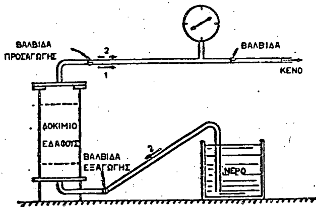
Σχήμα 2. Διάταξη απαερισμού και κορεσμού δοκιμίου.
