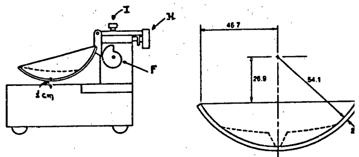
α) Μηχανική συσκευή ορίου υδαρότητας
