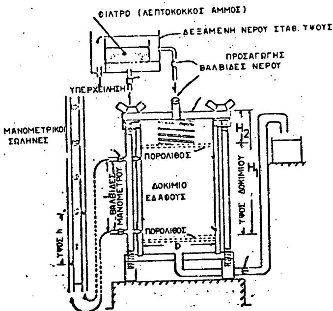
Σχήμα 1. Σχηματική παράσταση δοκιμής υδροπερατότητας σταθερού ύψους.
