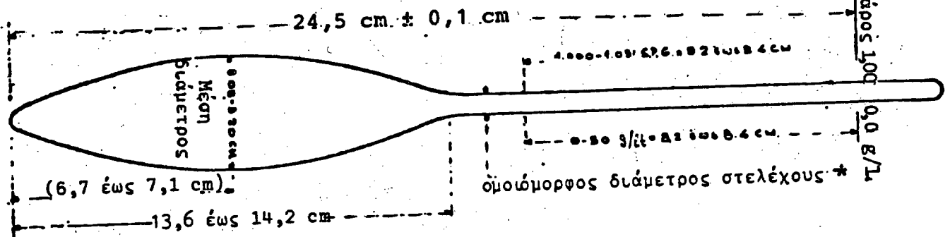
Σχήμα 2. Υδρόμετρο (Πυκνόμετρο).
