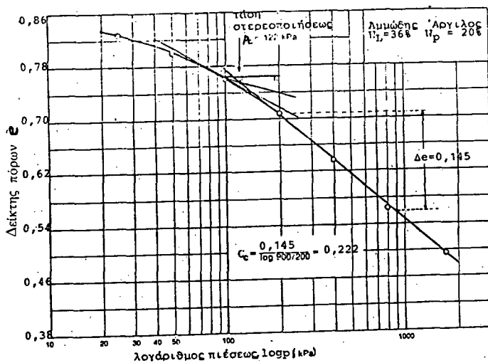
Σχήμα 5. Μεταβολή του δείκτη πόρων με τον λογάριθμο της κατακόρυφης τάσεως.
