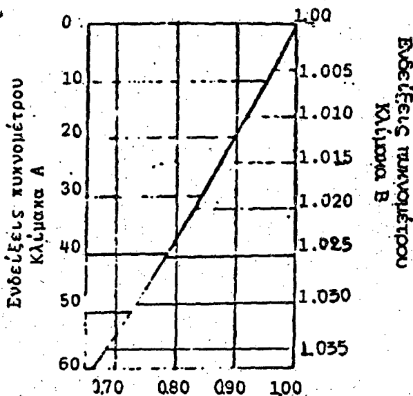
Σχήμα 3. Συντελεστής διορθώσεως K_L , για την ανύψωση του πυκνομέτρου εντός του αιώρηματος
