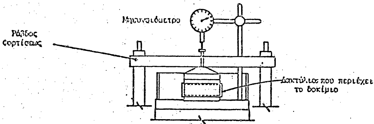
(α) Συσκευή Στερεοποίησης - Διάταξη Φορτίσας
