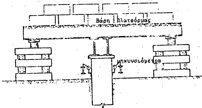
Σχ. 3. Διάταξη επιβολής φορτίου απευθείας στον πάσσαλο με ζυγισμένη πλατφόρμα.
